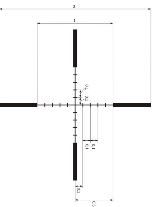
Рисунок 33 – Прицельная сетка (размер в м/100м дистан-
