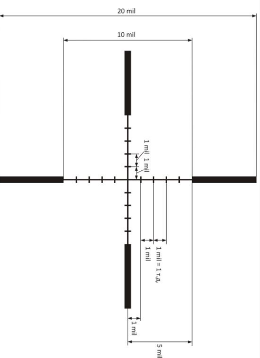
Рисунок 32 – Прицельная сетка (размер в миллирадианах
